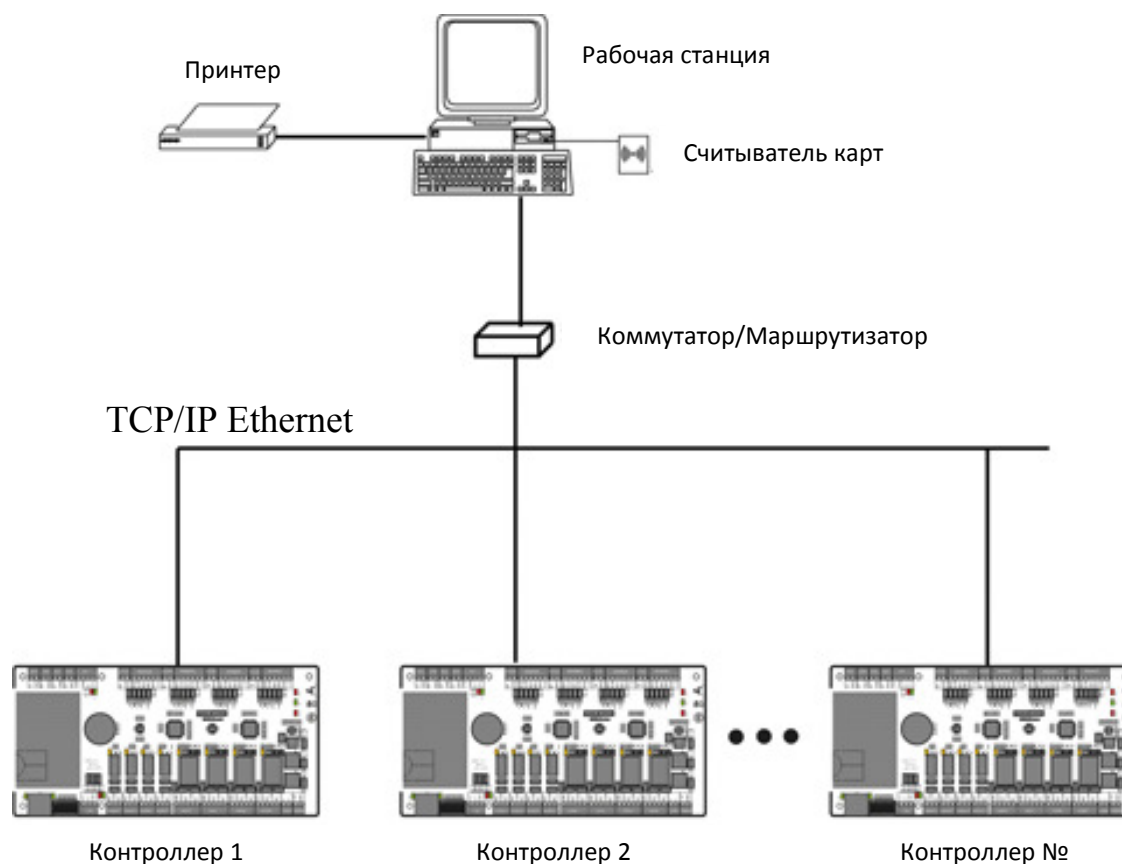
Топология TCP/IP
