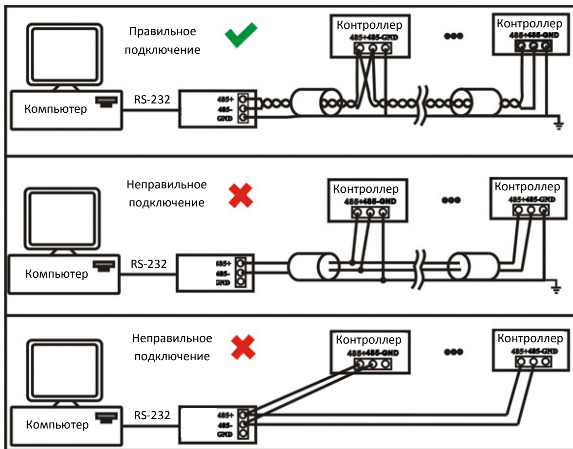
Топология RS-485
