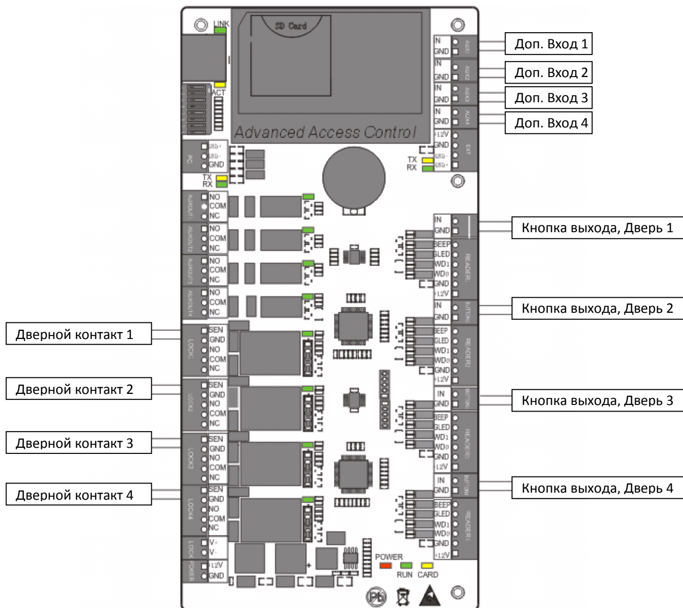
Подключение дверных контактов, кнопок выхода и дополнительных входов контроллера ST-NC440
