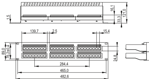
Рисунок 8 – PP48-2UC5EU-D05-1
