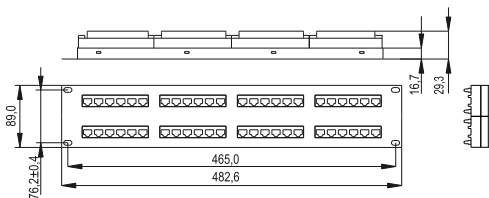
Рисунок 4 – PP48-2UC5EU-D05, PP48-2UC5EU-D05L
