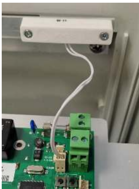
Рисунок 3.6.2 - Датчик вскрытия на корпусе коммутатора
