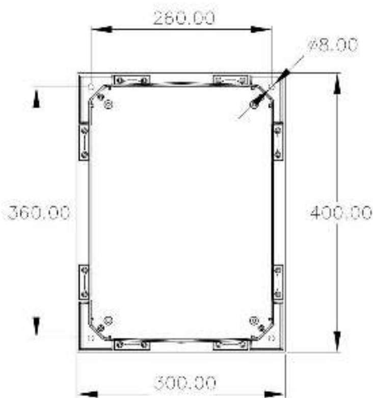
Рисунок 7.1 - Разметка крепления
