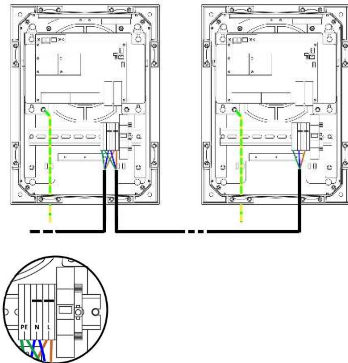
Рисунок 7.4 - Схема подключения цепочки коммутаторов
