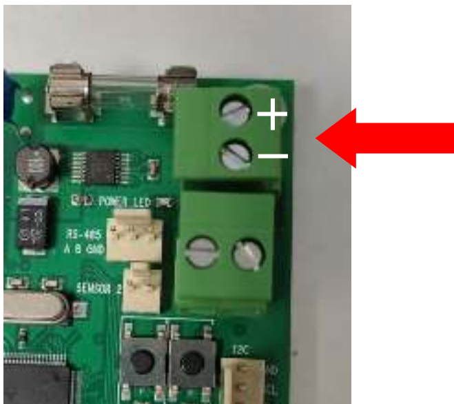
Рисунок 3.4.4 – Разъем для подключения альтернативного электропитания
