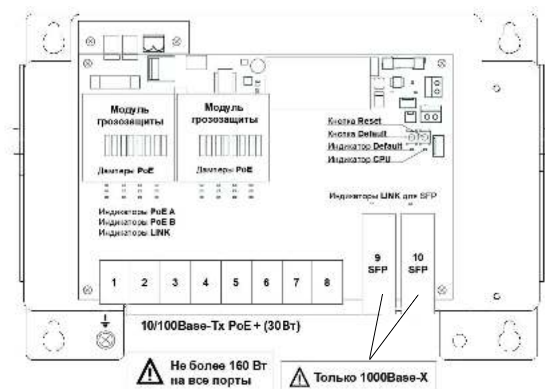
Рисунок 3.4.2 - Расположение элементов PSW-2G8F+Box
