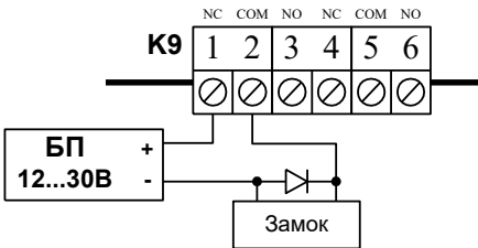
Пример 1. Подключение электромагнитного замка (однодверный режим)
