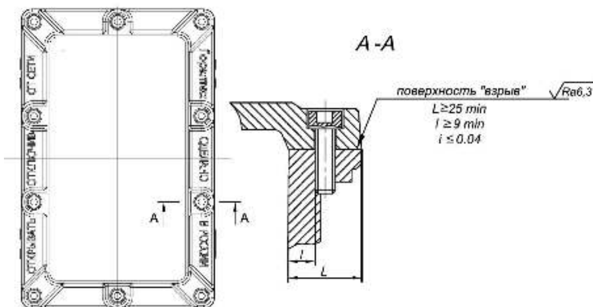
Рисунок 1.5а – Обеспечение взрывозащиты для оболочки
