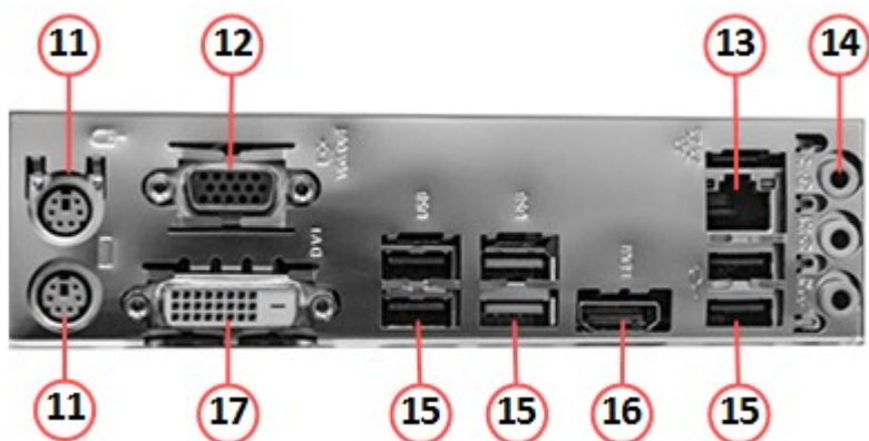
Рисунок 3. Разъемы на задней панели
