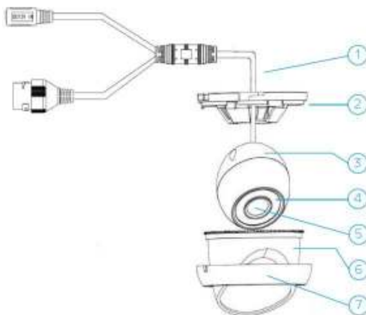
Рисунок 2. Устройство камеры
