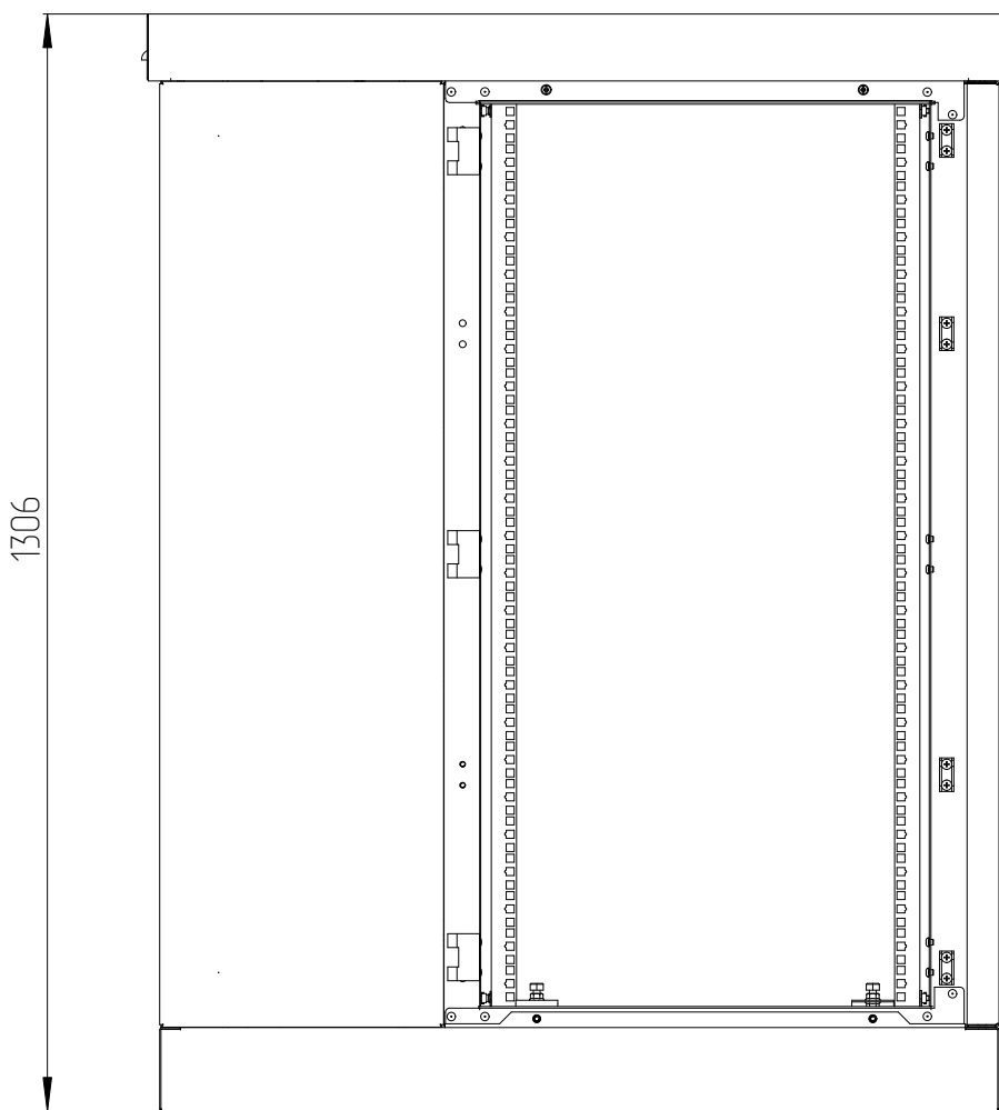
ШТВ-2-30.10.9-4.3А3
