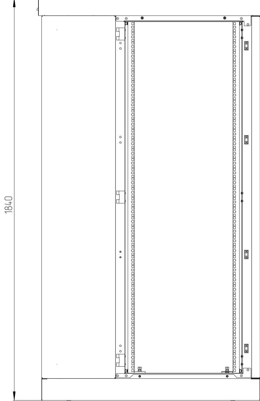
ШТВ-2-36.10.9-4.3А3
