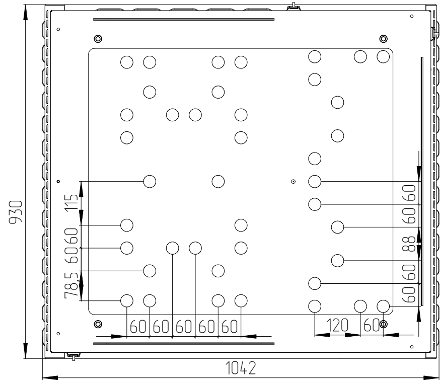
Вид снизу и габариты по крыше
