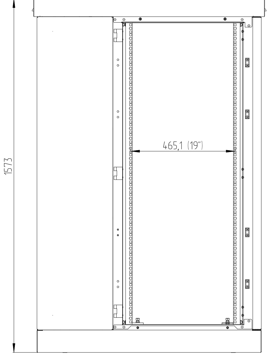
ШТВ-2-30.10.9-4.3А3
