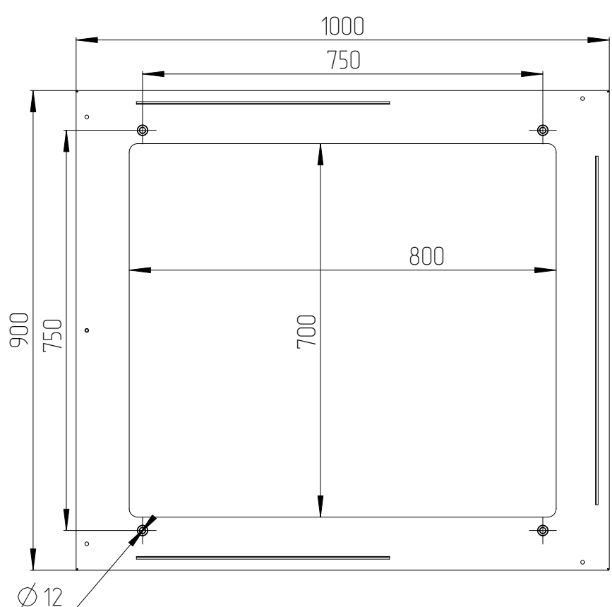
Цоколь базовый (высотой 100мм)
