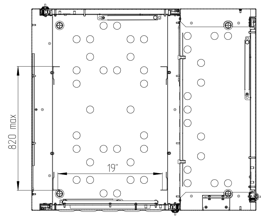
Сечение шкафа, каб. вводы
