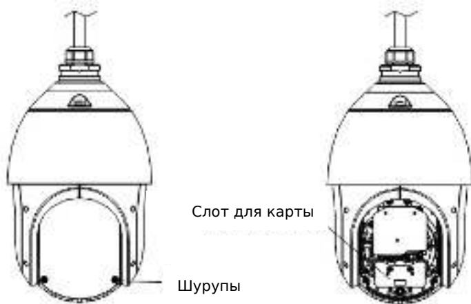
Рисунок 2-2 Установка SD-карты
