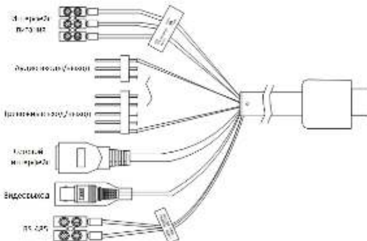
Рисунок 1-2 Кабели скоростной поворотной камеры
