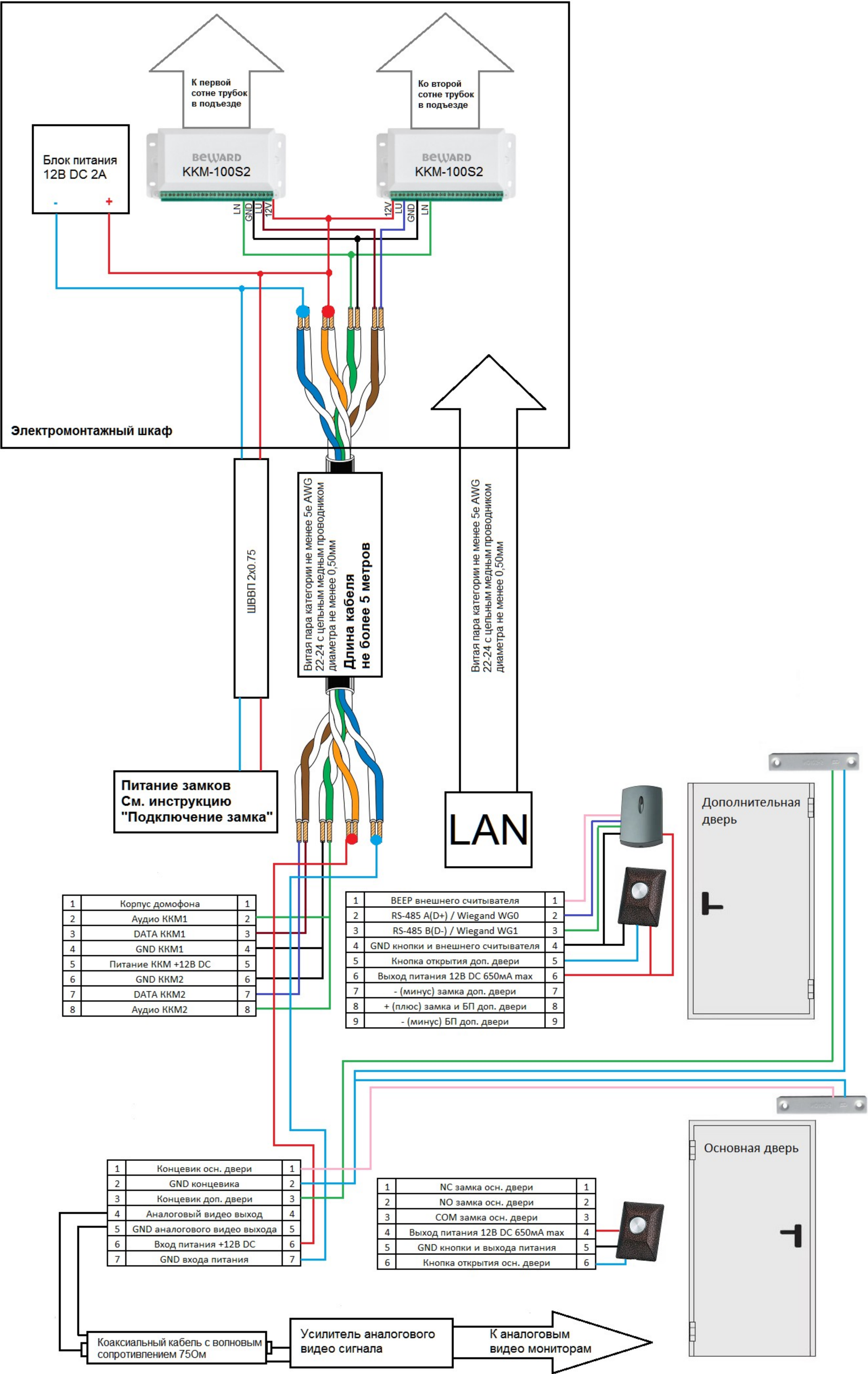
Схема подключения DKS151x4 DKS20211 (длина кабеля не более 5 метров)
