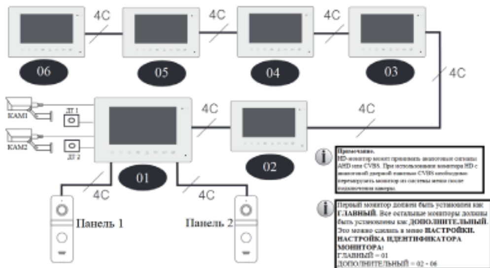
Схема подключения
