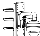
DS-1275ZJ-SUS Кронштейн для установки на столб (стойку)
