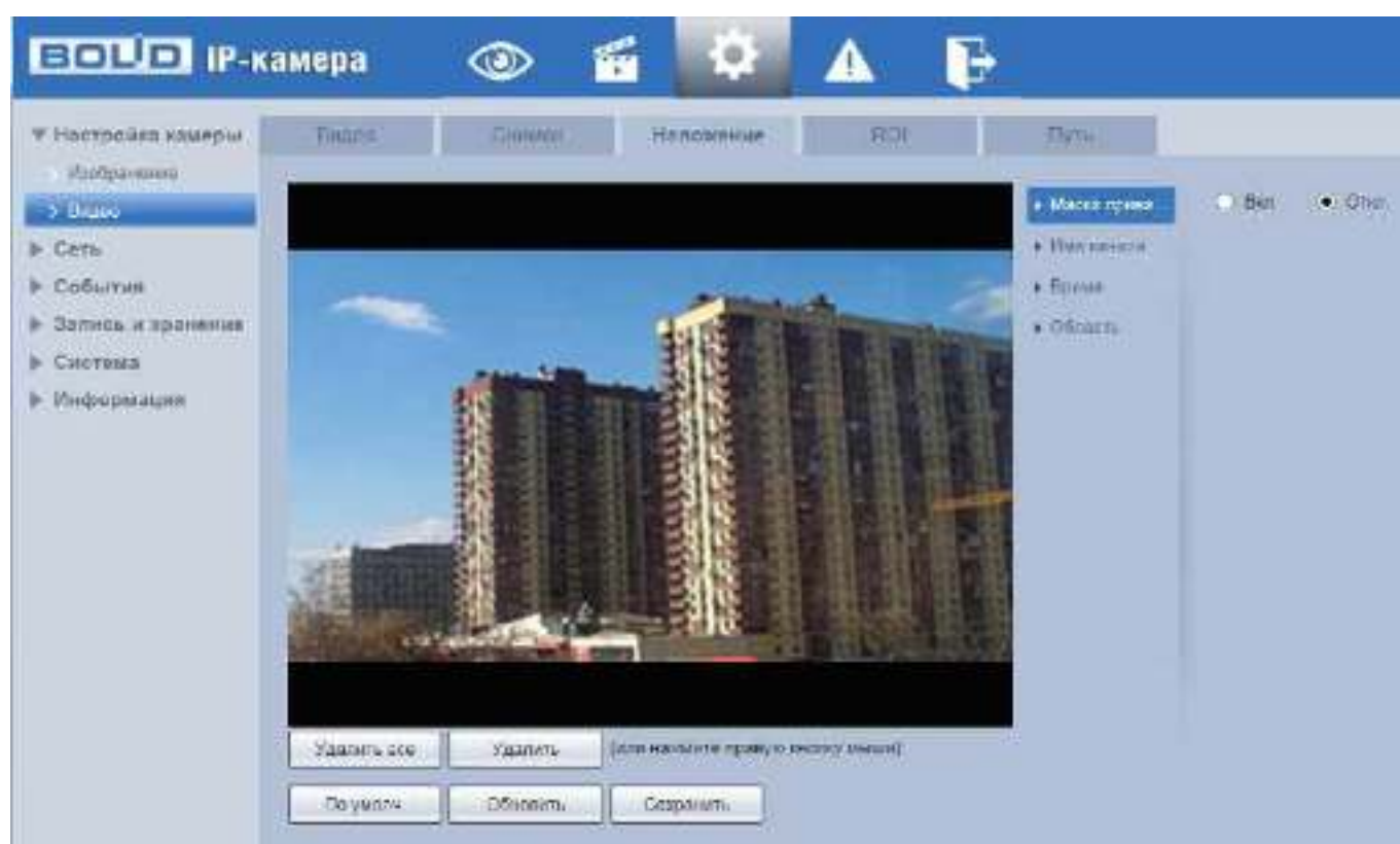
Рисунок 7.40 – Вкладка «Наложение»
