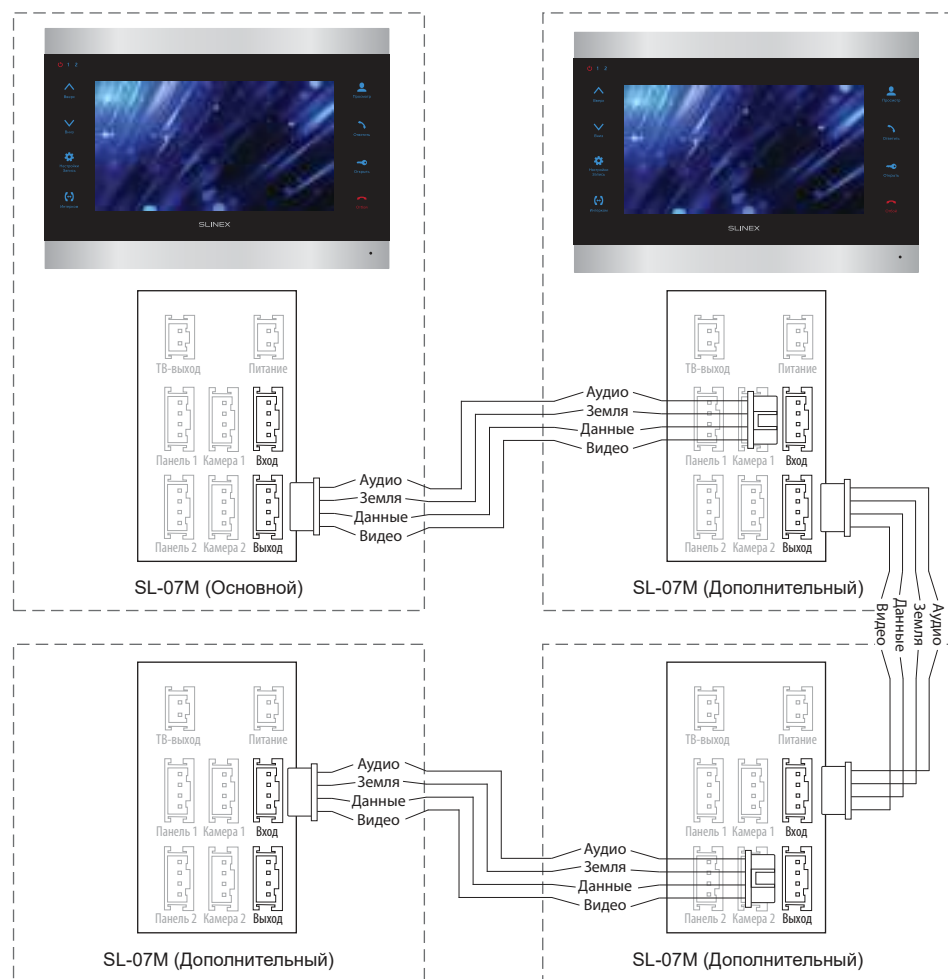
Схема 2. Подключение системы домофонов SL-07M.
