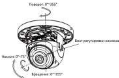
Рисунок 2-8 Регулировка угла наблюдения камеры III и IV типов
