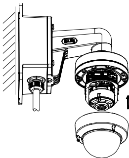
Рисунок 2-18 Установка купола
