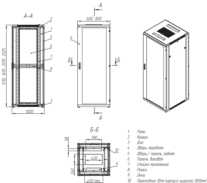
Рисунок 1. Габаритные размеры и внешний вид шкафа
