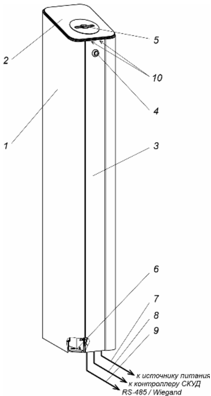
Рисунок 2. Устройство картоприемника:
