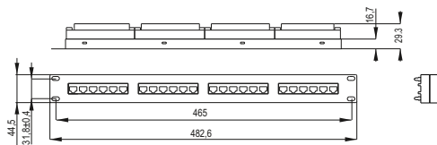
Рисунок/Figure 1 - PP24-1UC6U-D05
