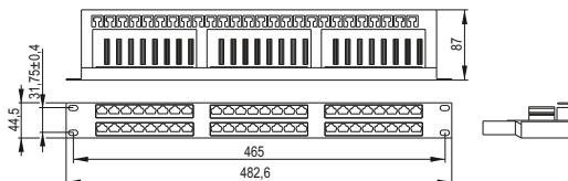
Рисунок/Figure 3 – PP48-1UC6U-D05H
