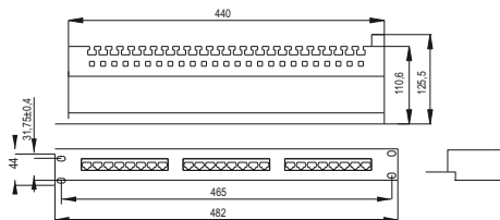
Рисунок/Figure 6 - PP24-1UC6S-D05
