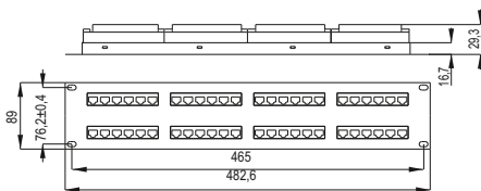
Рисунок/Figure 4 – PP48-2UC6U-D05, PP48-2UC6U-D05-1
