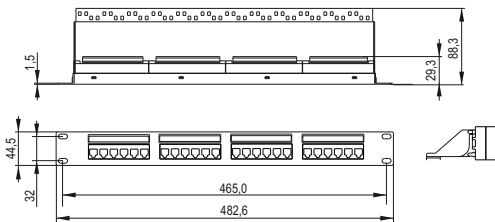
Рисунок/Figure 2 – PP24-1UC6U-D05-1
