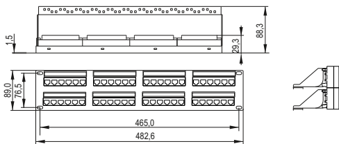
Рисунок/Figure 5 – PP24-D05UC06S-D05H
